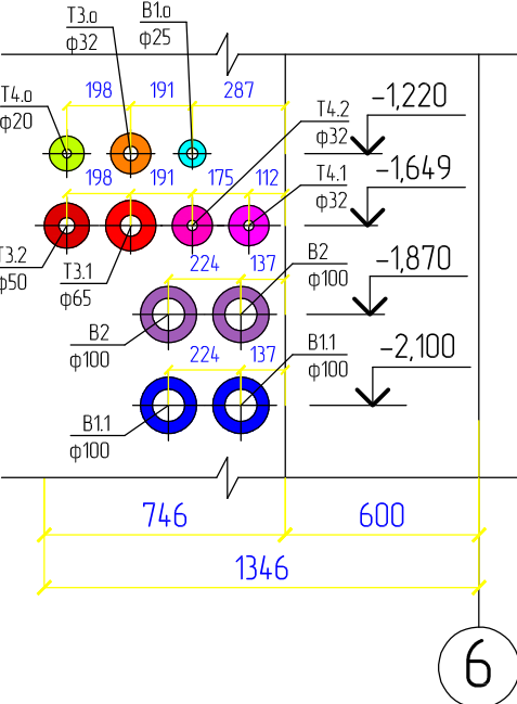
Разрез А-А
